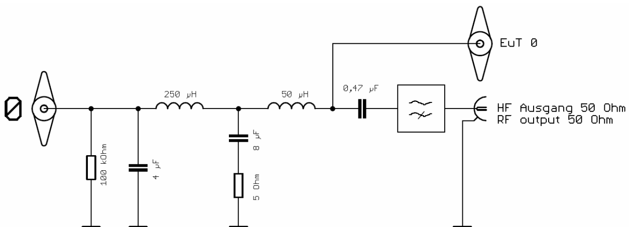
Abb. 1 Schaltplan NNLK 8122 Fig. 1 Schematics NNLK 8122
