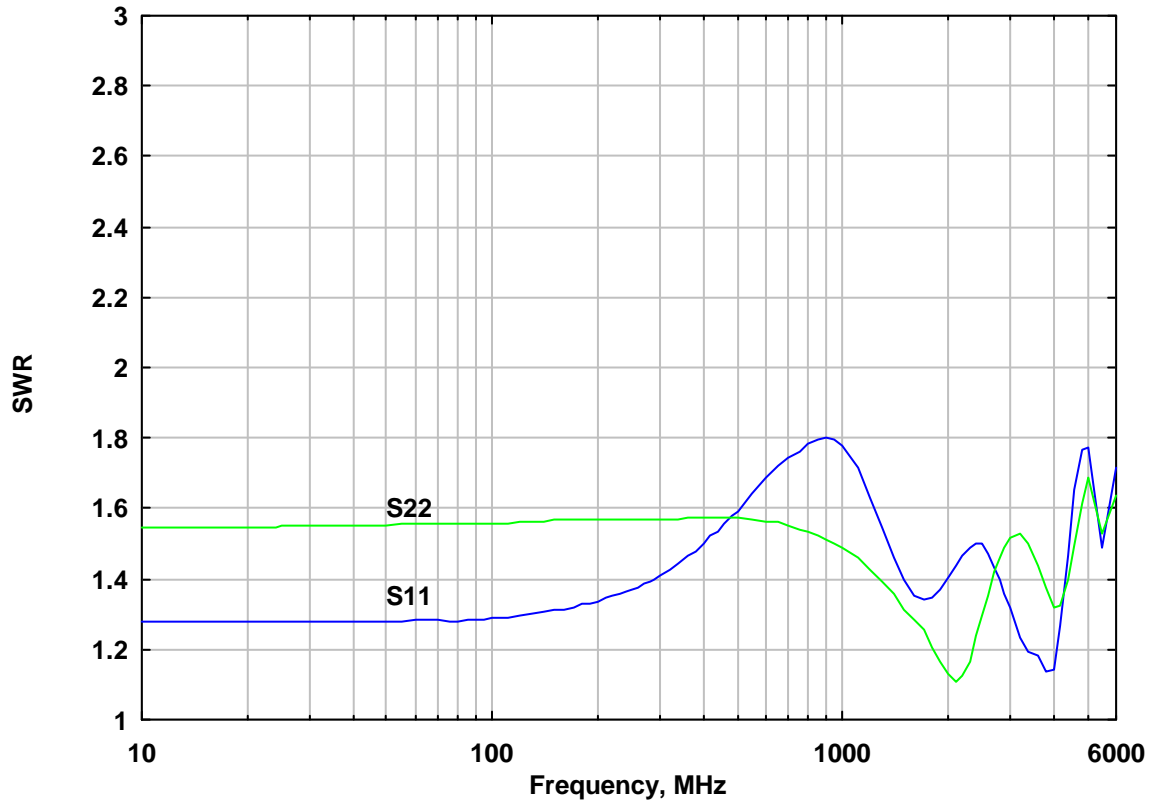
Eingangsanpassung S11, Ausgangsanpassung S22 Input Match S11, Output Match S22
