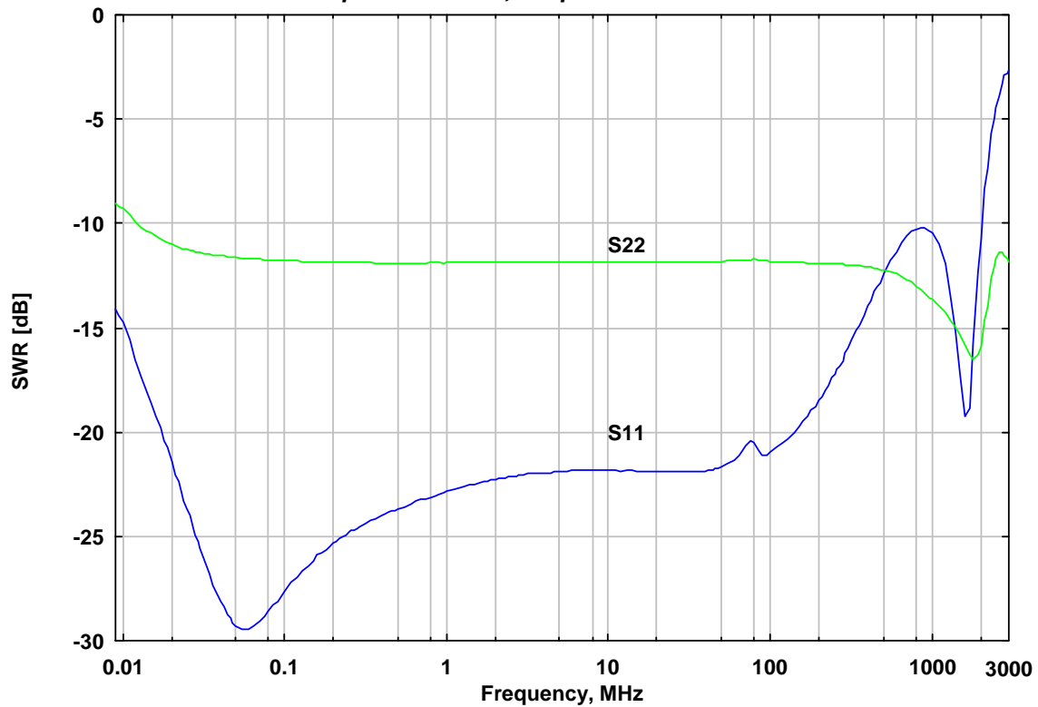
Eingangsanpassung S11, Ausgangsanpassung S22 Input Match S11, Output Match S22
