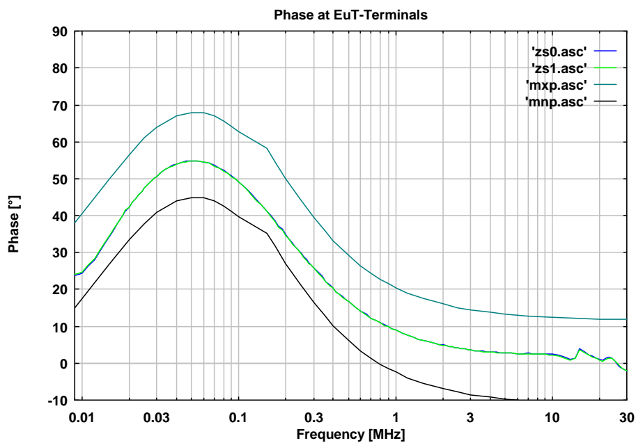
Abb. 8 Phase an den Prüflingsklemmen (SCHUKO), BNC mit 50 Ω Abschluss Phase at the connector for DuT (Schuko), BNC terminated with 50 Ω
