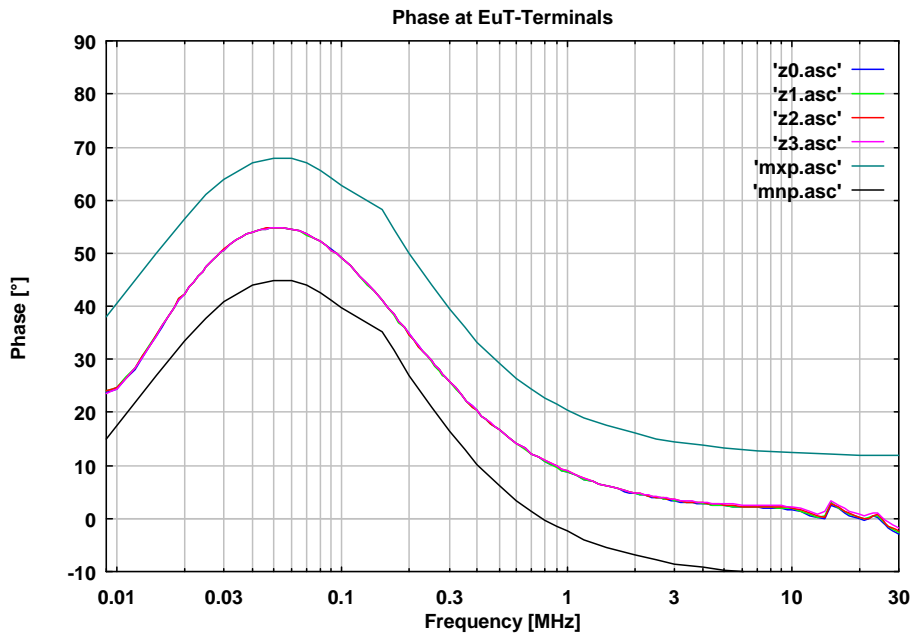
Abb. 5 Phase an den Prüflingsklemmen (CEKON), BNC mit 50 Ω Abschluss Phase at the connector for DuT (CEKON), BNC terminated with 50 Ω
