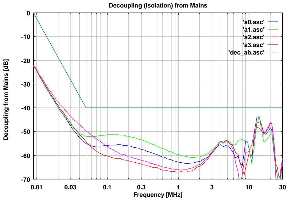
Abb. 9 Entkopplung vom Speisernetz (CEKON-Prüflingsklemmen), BNC mit 50 Ω Abschluss Decoupling from supply net (CEKON), BNC terminated with 50 Ω
