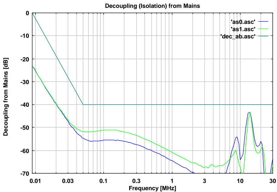
Abb. 10 Entkopplung vom Speisernetz (SCHUKO-Prüflingsklemmen), BNC mit 50 Ω Abschluss/ Decoupling from supply net (Schuko), BNC terminated with 50 Ω
