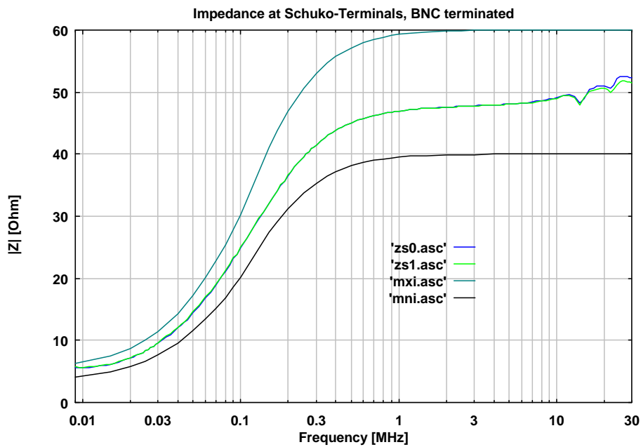
Abb. 7 Impedanz an den Prüflingsklemmen (SCHUKO), BNC mit 50 Ω Abschluss Impedance of connector for DuT (Schuko), BNC terminated with 50 Ω
