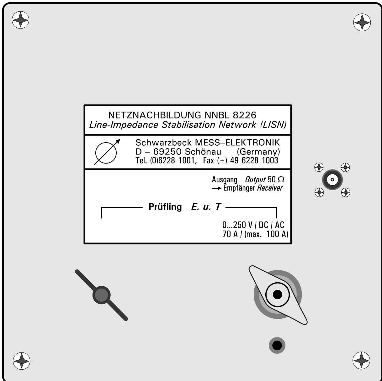
Netznachbildung LISN NNBL 8226
