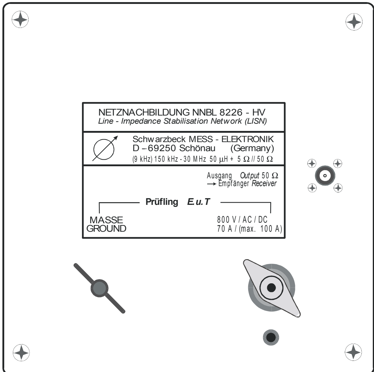
Netznachbildung LISN NNBL 8226 - HV
