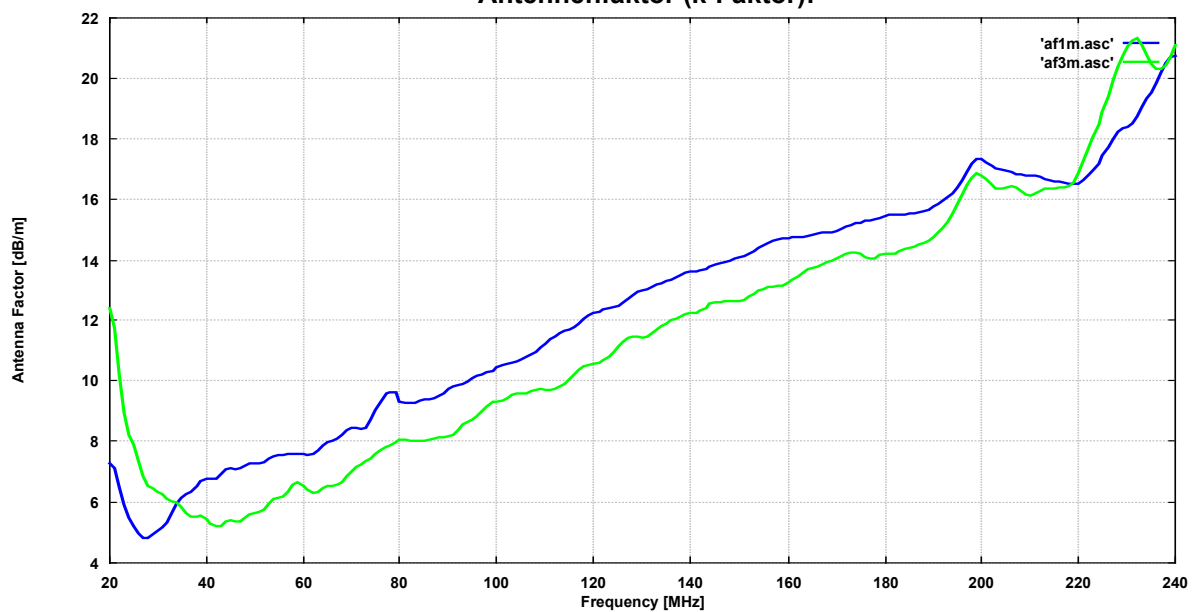
Antennenfaktor (k-Faktor):
