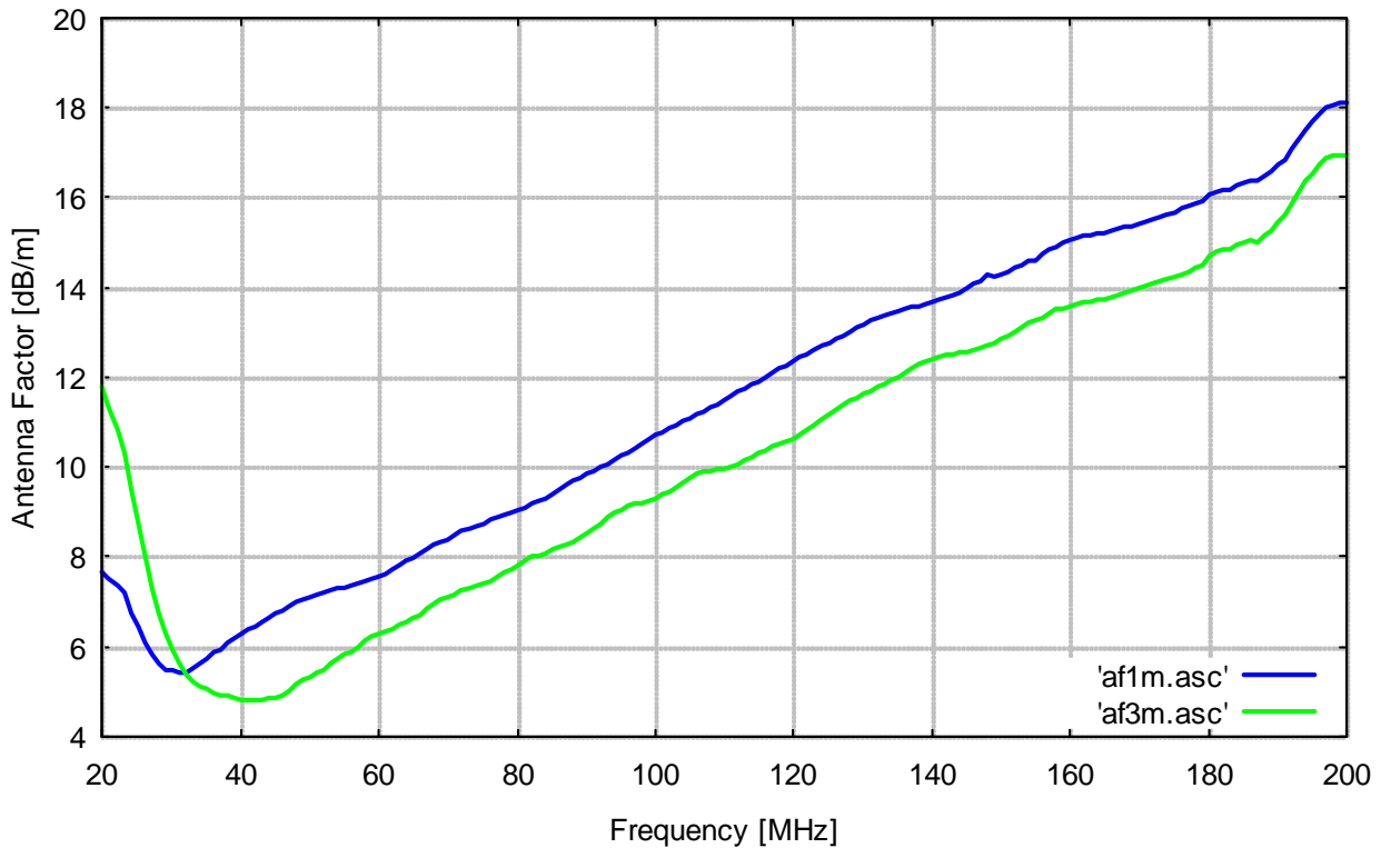
Antennen-Wandlungsmaß
