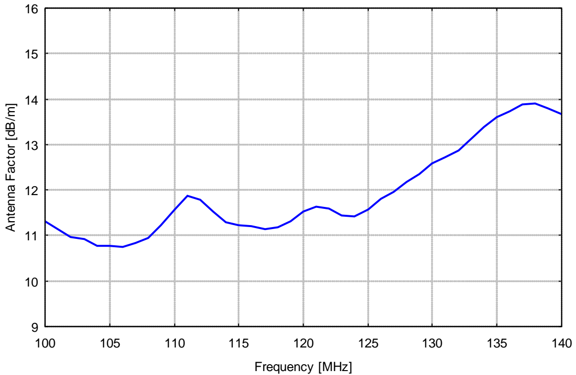
Antennen-Wandlungsmaß
