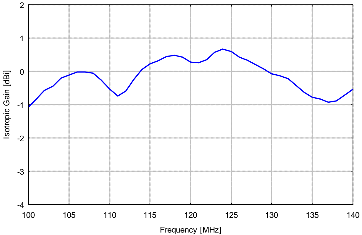
Isotropgewinn
