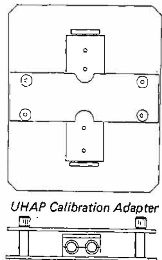
UHAP Kalibrier-Adapter (UHF)
