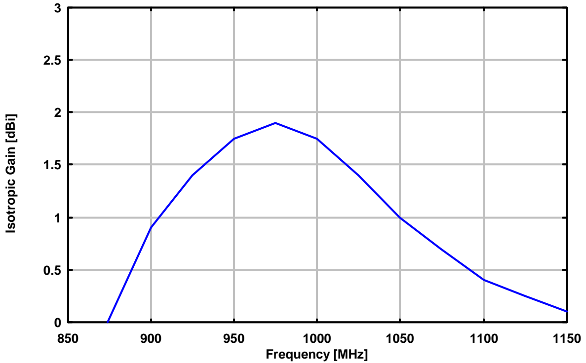
Isotropgewinn, Kurzschlußschieber entfernt UHA 9125 D LE=140 mm, Short=Removed
