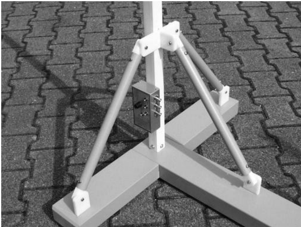
Teilansicht mit Koaxialumschalter Detail View with Coaxial Switching Unit
