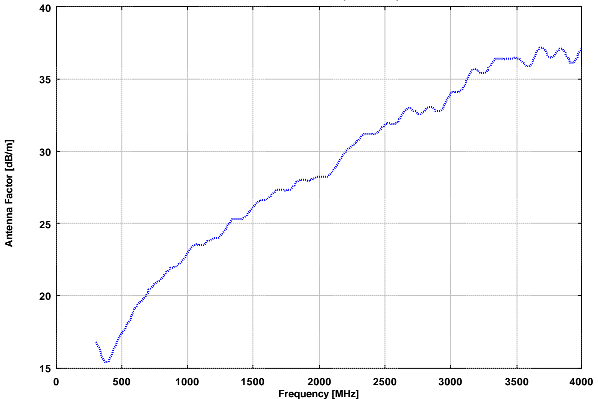
Antennenfaktor (k-Faktor):
