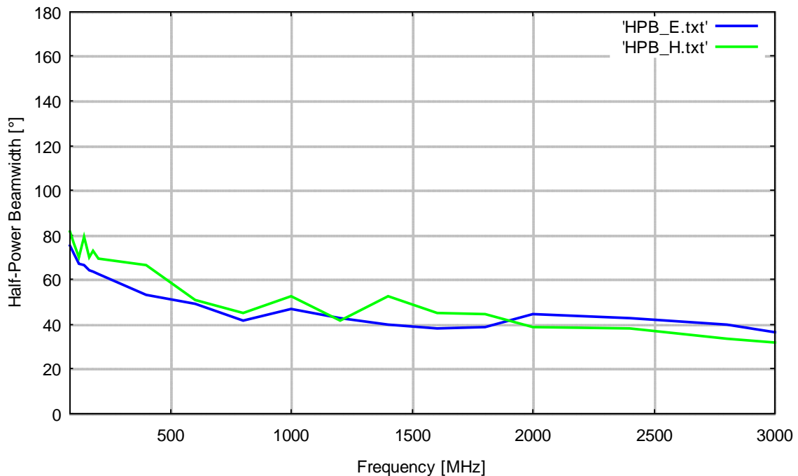
3 dB Öffnungswinkel [°]
