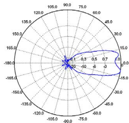
H-Ebene / H-Plane 1.4 GHz
