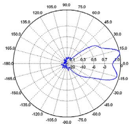
E-Ebene / E-Plane 1.4 GHz
