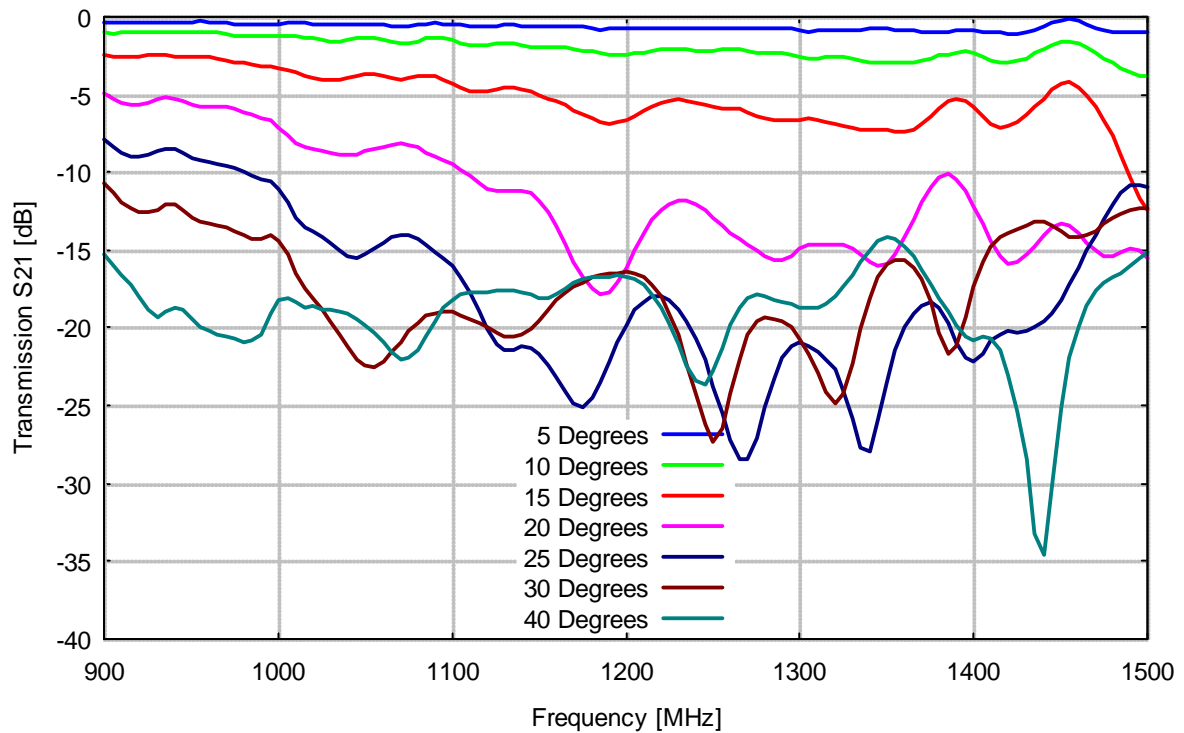
H-plane
